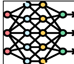
統合解析
