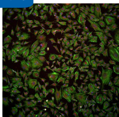
形態解析
