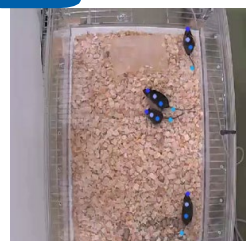
行動解析
